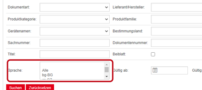
Fig. 12: Limbă - Selectare
