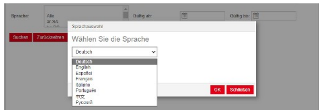
Abb. 6: Auswahlfenster Sprachauswahl
