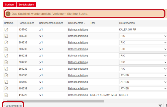
Fig. 13: Sökgräns: 100 element
