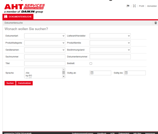
Joonis 1: Dokumendiotsing
