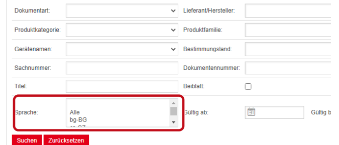
Fig. 12: Språk - Valg
