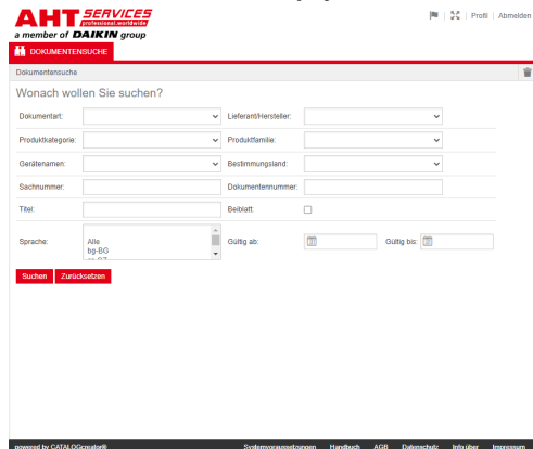
ábra 1: Dokumentumok keresése
