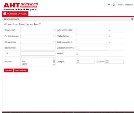
Fig. 1: Dokumentsøk
