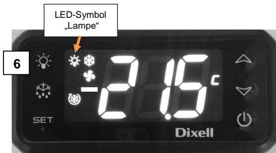
Abb. 3.1 Reglertyp DIXELL Bedienelemente und Display- anzeigen (Symboldarstellung)
